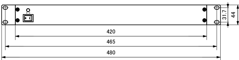
正面図
