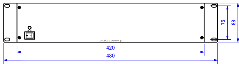
正面図
